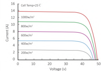
ВАХ при різній інсоляції (LR5-72HPH-530M)
