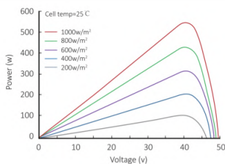
ВАХ при різній температурі (LR5-72HPH-530M)
